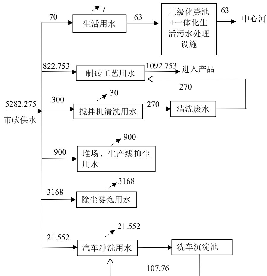
图 2-1 项目水平衡图（单位：m³/a）
